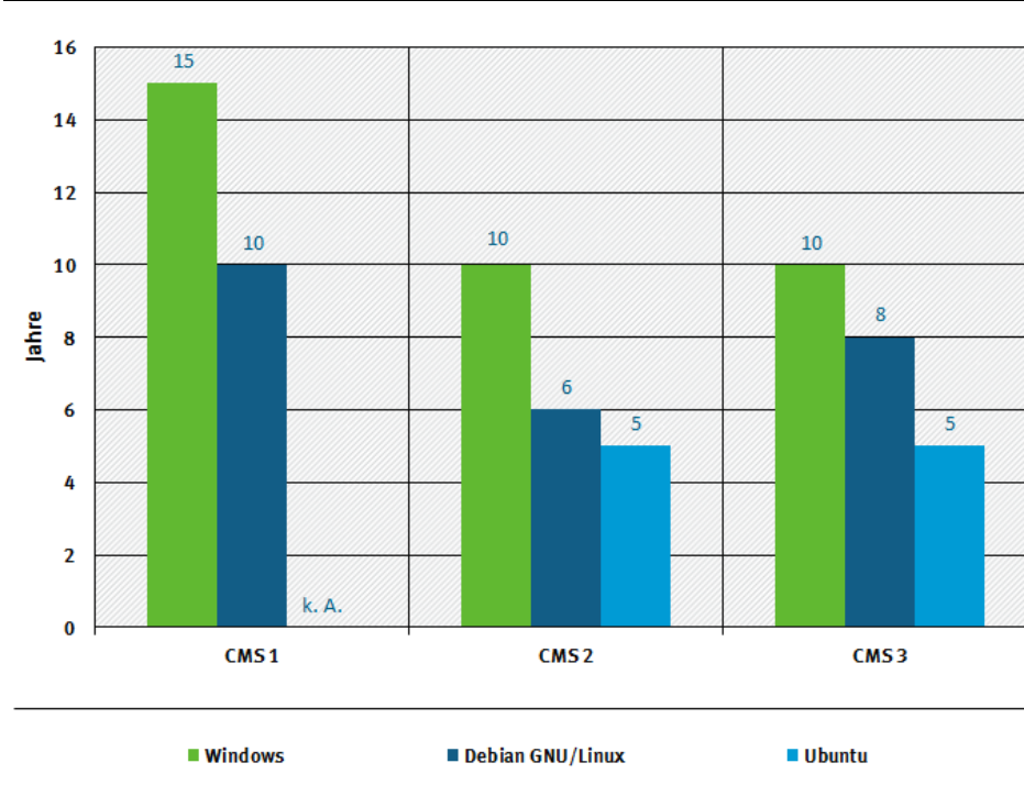
Abbildung 24: Abwärtskompatibilität der Content Management Systeme nach Betriebssystem
