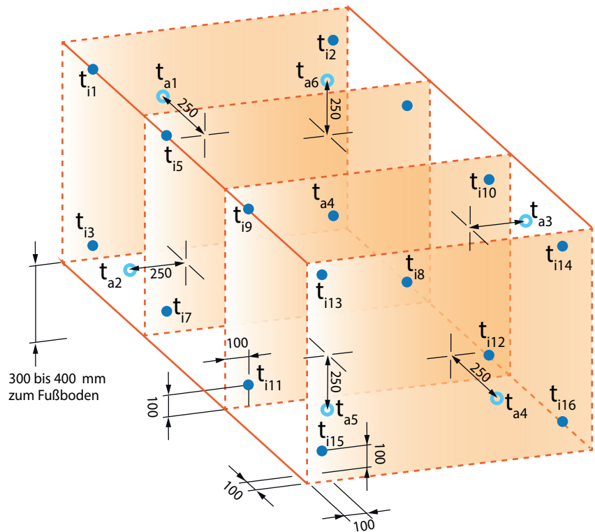
Bild 1: Position der Temperaturmessfühler nach DIN EN 1886 (Abmessungen in mm). Bild: Schiller-Krenz
